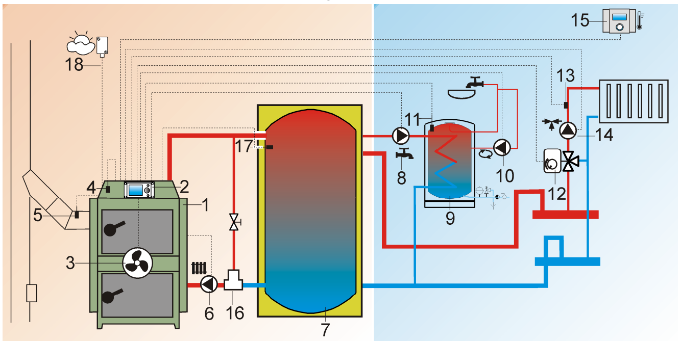
Obr. 18 Schéma s akumulční nádrží – bez dodatkových modulů , kde: 1 - kotel, 2 – regulátor , 3 – ventilátor, 4 – čidlo teploty kotle, 5 – čidlo teploty spaliny, 6 – čerpadlo kotle, 7 – akumulace, 8 – čerpadlo TUV, 9 – zásobník TUV, 10 – čerpadlo cirkulace TUV, 11 – čidlo TUV, 12 – pohon směšovače, 13 – čidlo směšovače, 14 – čerpadlo směšovače, 15 – pokojový panel SPARKSTER s funkcí termostatu, 16 – termostatický, směšovací ventil pro ochrnu zpátečky, nebo Laddomat, 17 – horní čidlo akumulace, 18 – venkovní čidlo teploty
