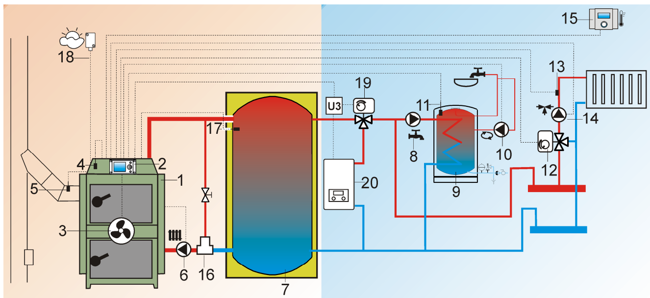
Obr. 20 Schéma s akumulční nádrží – s rezervním kotlem , kde: 1 - kotel, 2 – regulátor, 3 – ventilátor, 4 – čidlo teploty kotle, 5 – čidlo teploty spalin, 6 – čerpadlo kotle, 7 – akumulace, 8 – čerpadlo TUV, 9 – zásobník TUV, 10 – čerpadlo cirkulace TUV, 11 – čidlo TUV, 12 – pohon směšovače, 13 – čidlo směšovače, 14 – čerpadlo směšovače, 15 – pokojový panel SPARKSTER s funkcí termostatu, nebo běžný termostat 16 – termostatický, směšovací ventil pro ochrnu zpátečky, nebo Laddomat, 17 – horní čidlo akumulace, 18 – venkovní čidlo teploty, 19 – pohon přepínacího ventilu, 20 – rezervní kotel, U3 – modul pro rezervní kotel, popis v kpt. 28.14
